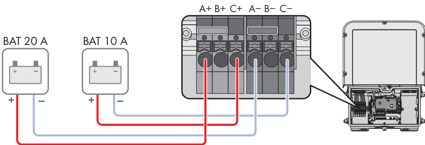
Imagen 19: Sinóptico de conexión para la conexión de 2 baterías, cuyas corrientes de carga/descarga se limitan de distinta forma
