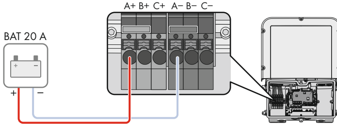
Imagen 20: Sinóptico de conexión para la conexión de una batería, cuya corriente de carga/descarga se limita a 20 A
