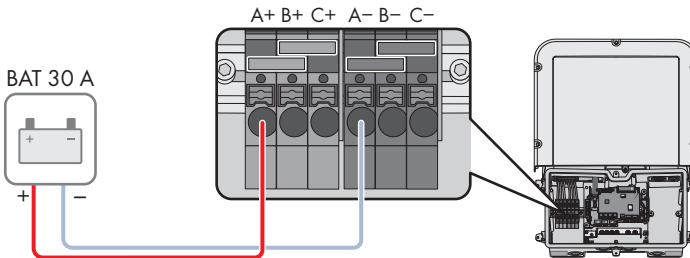
Imagen 21: Sinóptico de conexión para la conexión de una batería, cuya corriente de carga/descarga se limita a 30 A
