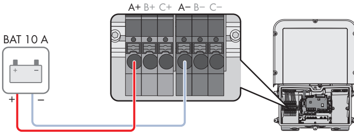
Imagen 16: Sinóptico de conexión para la conexión de una batería, cuya corriente de carga/descarga se limita a 10 A
