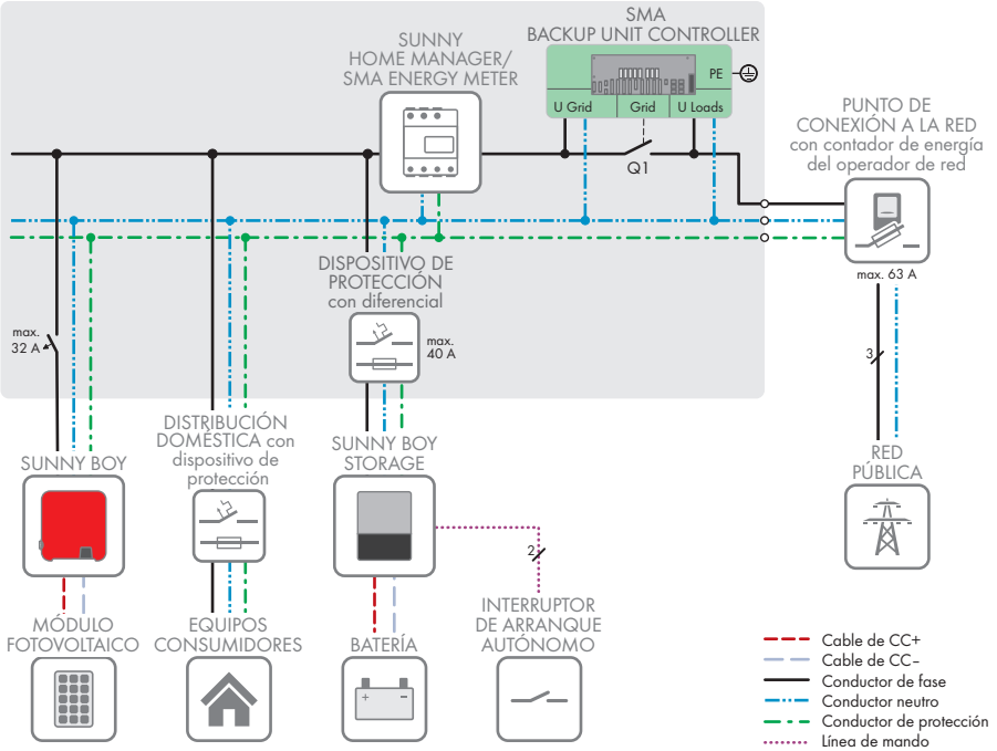
Imagen 6: Estructura del sistema del Flexible Storage System con función de alimentación de repuesto (ejemplo)
