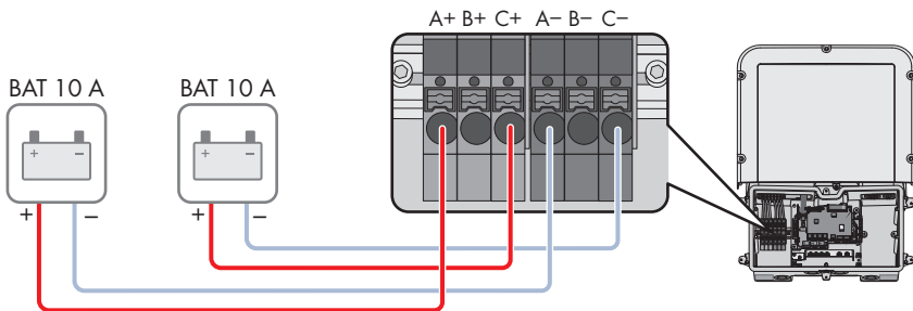
Imagen 17: Sinóptico de conexión para la conexión de 2 baterías, cuyas corrientes de carga/descarga se limitan a 10 A respectivamente
