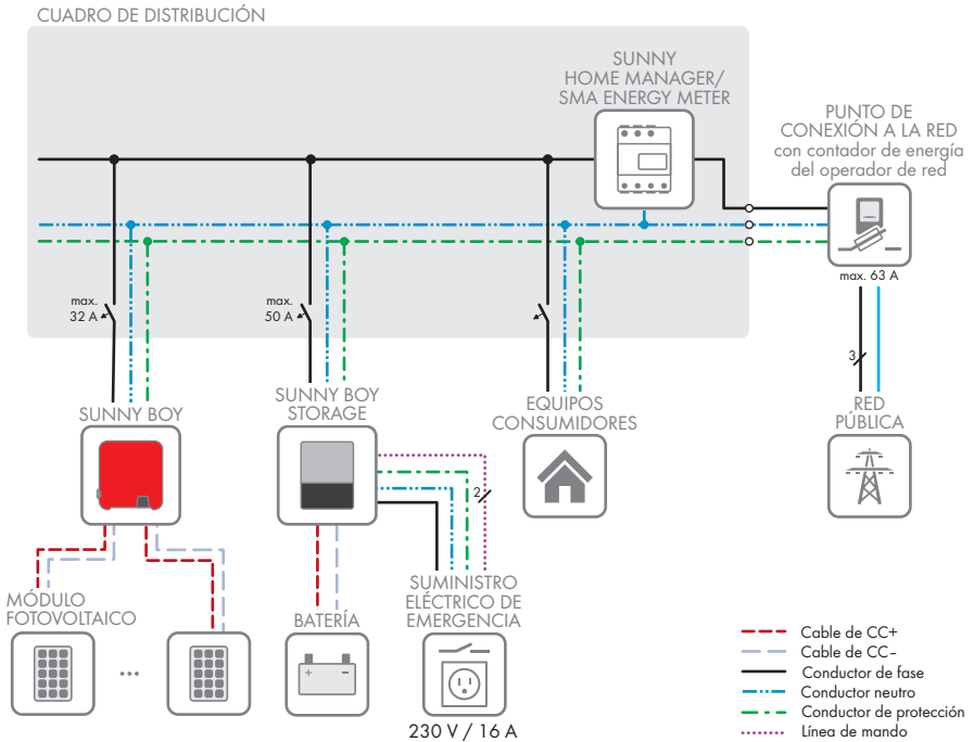
Imagen 5: Esquema de interconexión de un Flexible Storage System con interruptor y toma de pared para el funcionamiento de corriente de emergencia (ejemplo)
