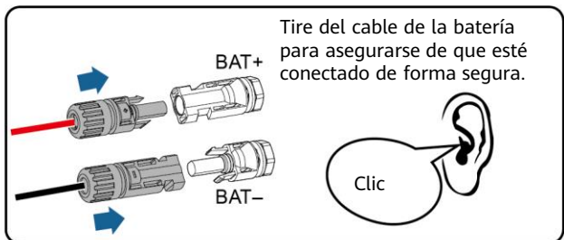
Bornes de la batería (BAT+/BAT-)
