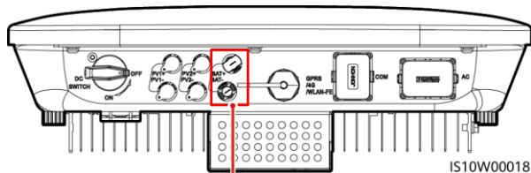
Bornes de la batería (BAT+/BAT-)
