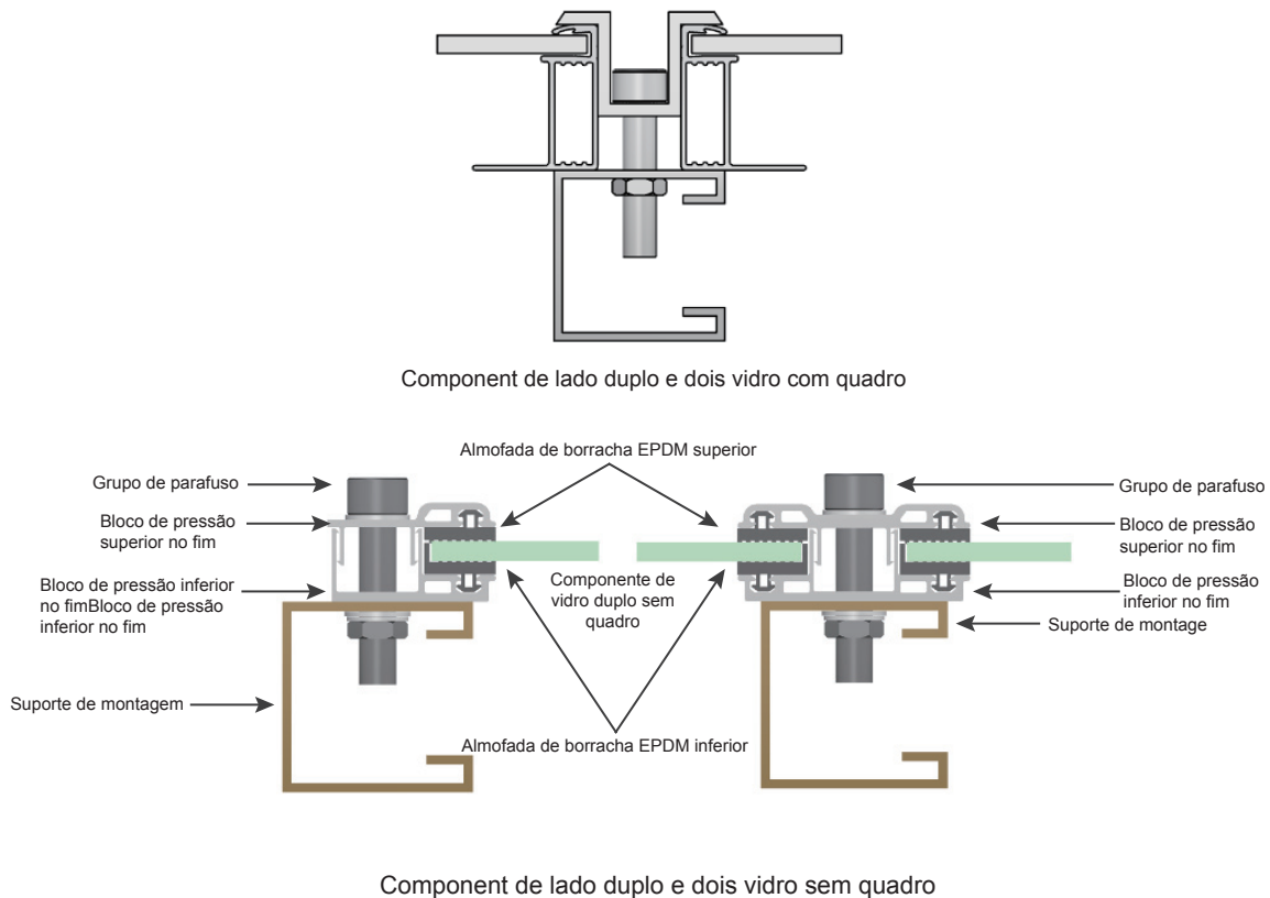
Figura 8 Diagrama de instalação dos fixações de montagem de componente de lado duplo
