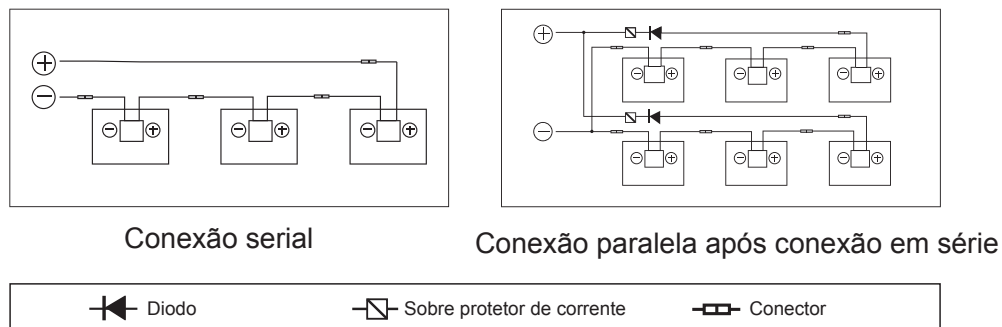
Figura 10 Diagrama elétrico do circuito conexão serial e conexão paralela
