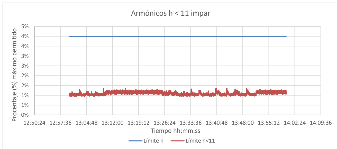
Figura 5. Armónicos h < 11 impar.
