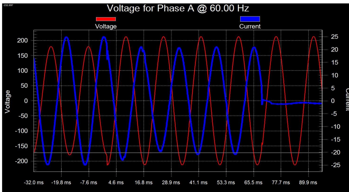
Figura 20 Tiempo de desconexión al 120% de tensión.
