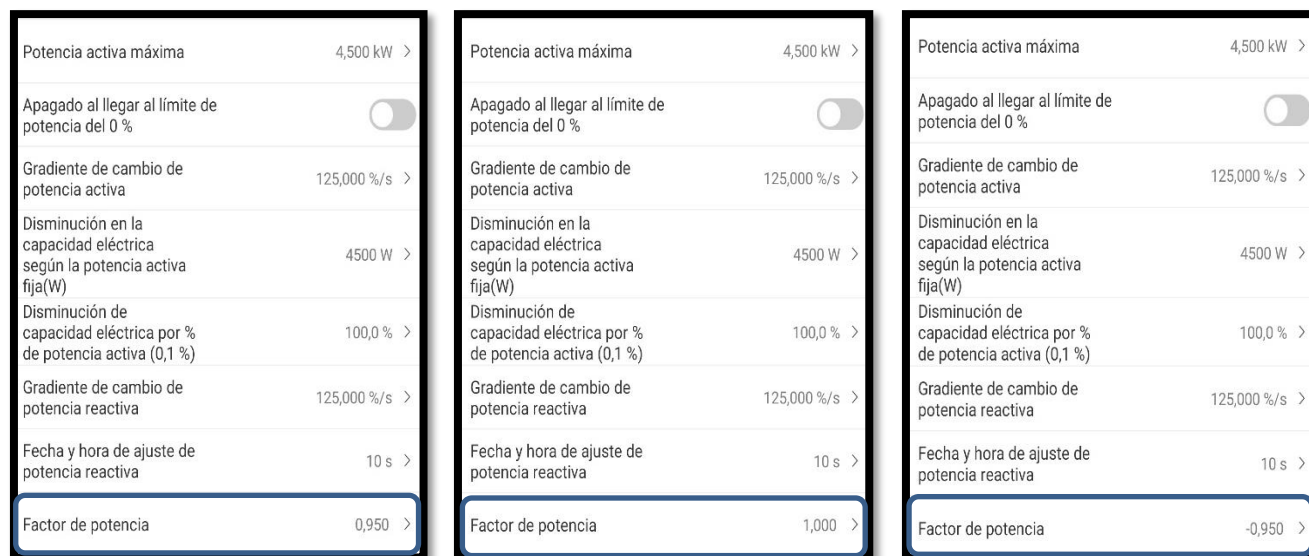
Figura 4. Configuración del factor de potencia en aplicación móvil "FusionSolar".
