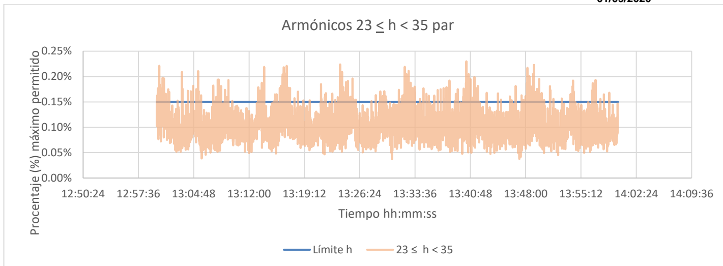
Figura 13. Armónicos 23 \leq h < 35 par.
