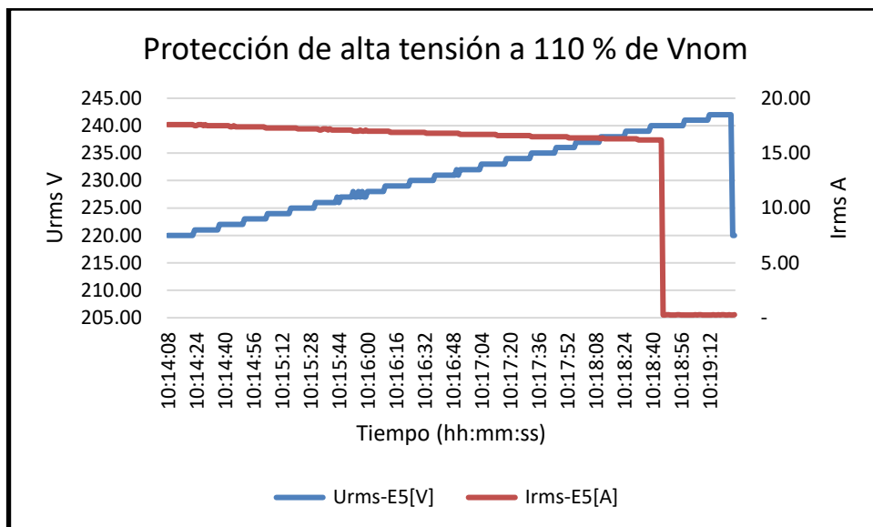
Figura 16. Desconexión por sobre tensión.
