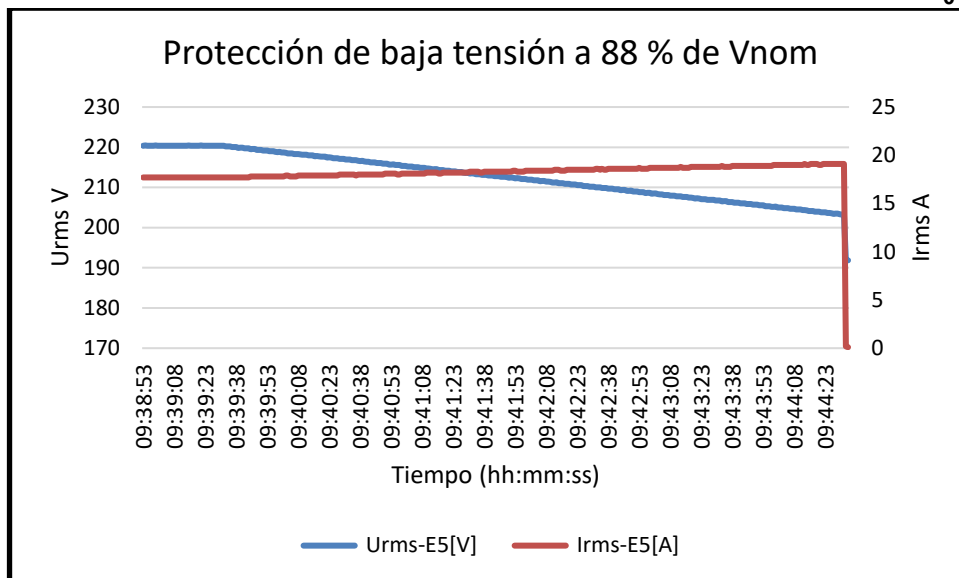
Figura 15. Desconexión por baja tensión.
