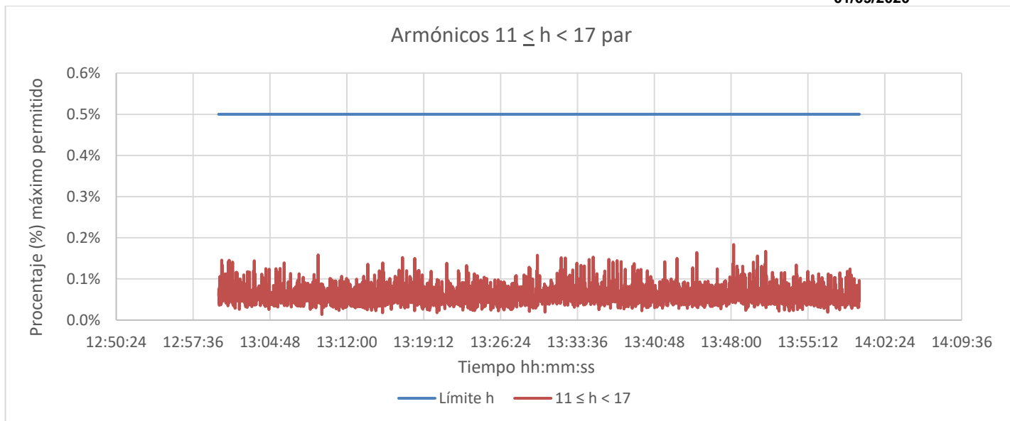
Figura 11. Armónicos 11 \leq h < 17 par.
