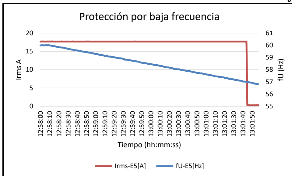
Figura 22. Disparo por Baja Frecuencia.
