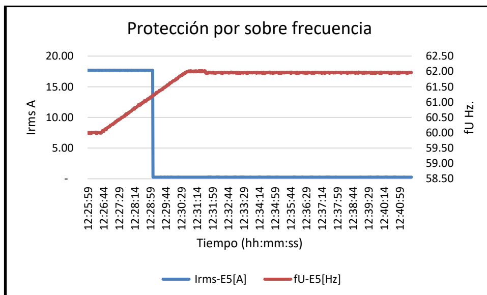
Figura 21. Disparo por Sobre Frecuencia.
