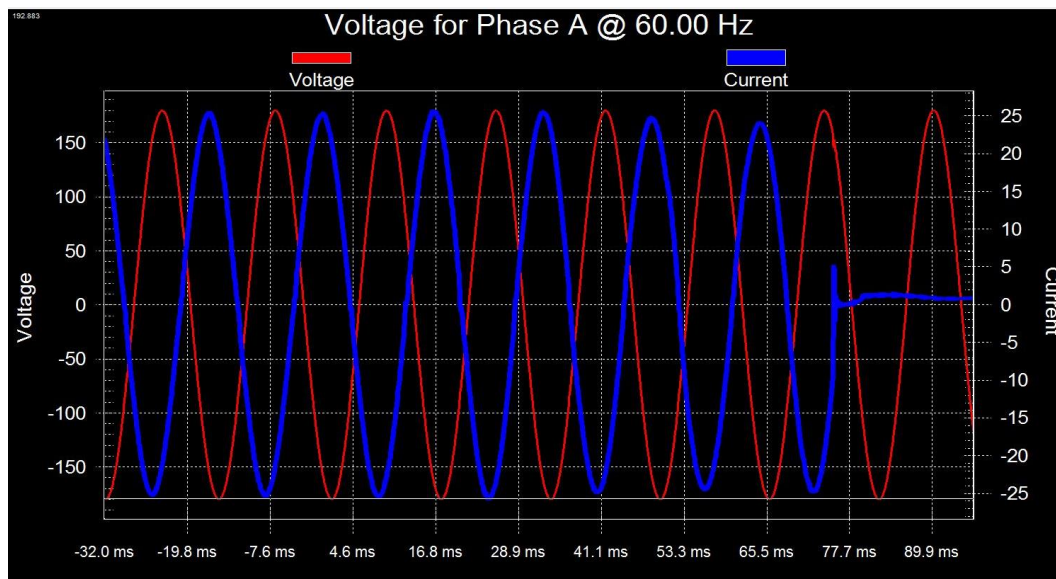
Figura 23. Tiempo de desconexión en alta frecuencia 61.2Hz
