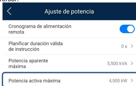
Figura 2. Programación mediante la App "FusionSolar".
