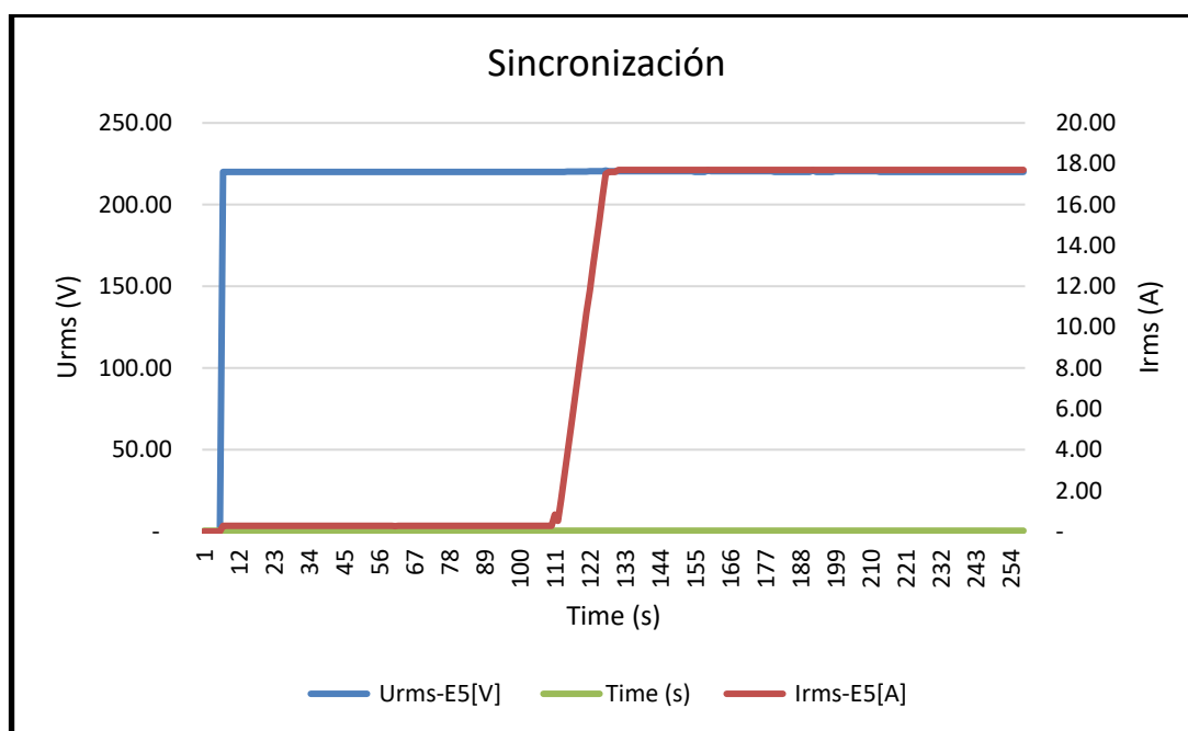
Figura 3. Gráfica de sincronización.
