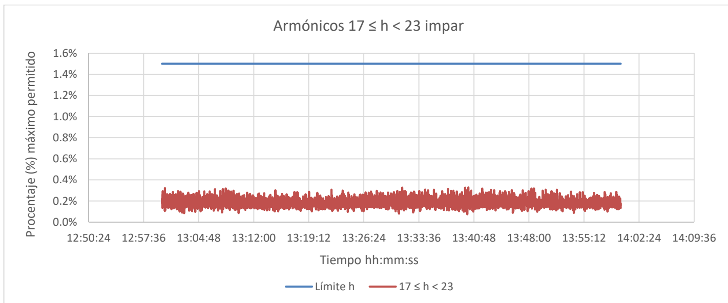
Figura 7. Armónicos 17 \leq h < 23 impar
