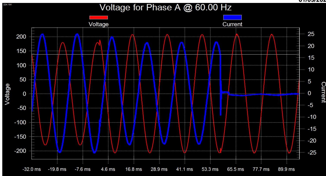
Figura 19 Tiempo de desconexión al 115% de tensión.
