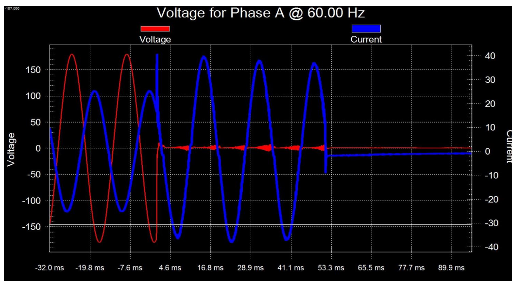
Figura 26. Gráfica de anti-isla.
