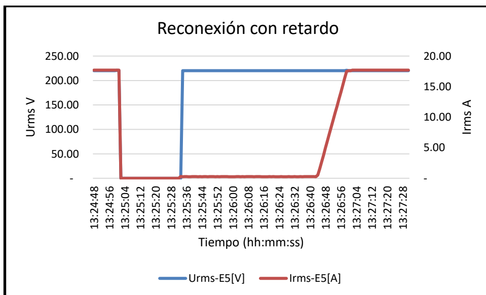
Figura 25. Gráfica de reconexión.
