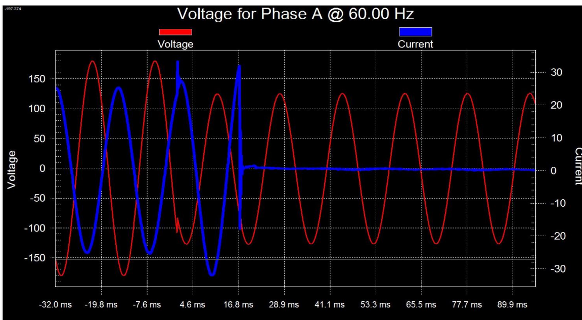
Figura 18. Tiempo de desconexión al 70 % de tensión.
