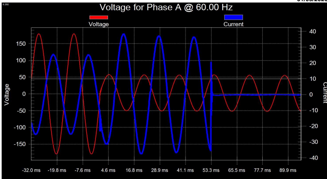
Figura 17. Tiempo de desconexión al 30 % de tensión.
