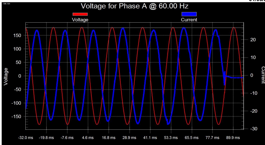
Figura 24. Tiempo de desconexión en baja frecuencia 57Hz.
